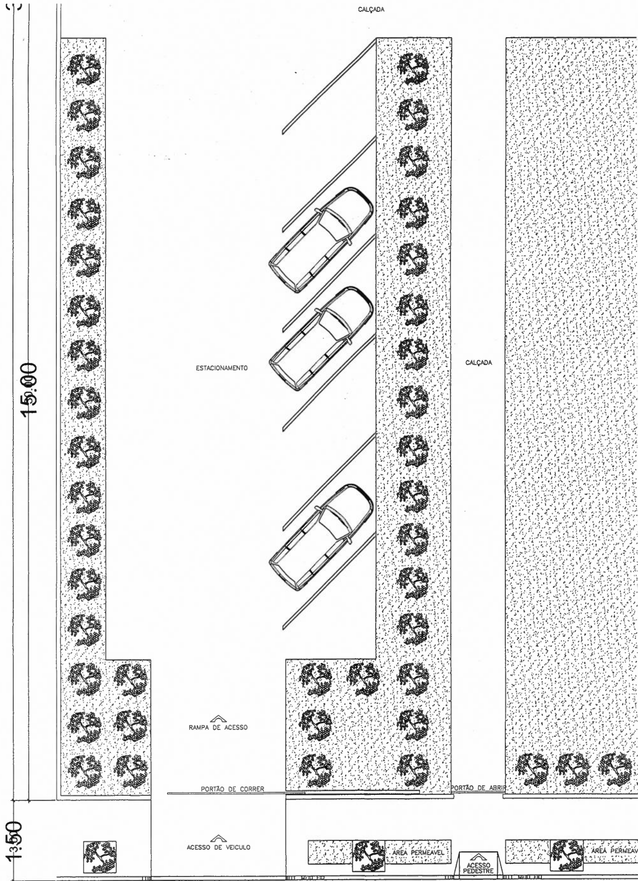
IMPLANTAÇÃO ESCALA: 1:100
