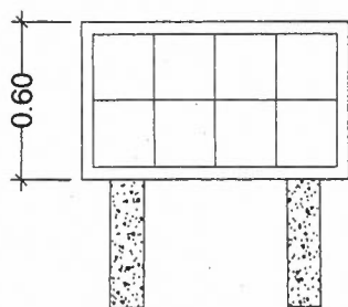
ELEVAÇÃO
